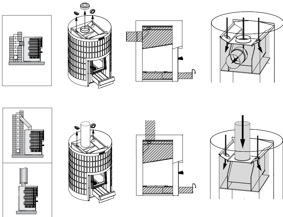
15. attēls. Pirts sildītāja slaucīšana
