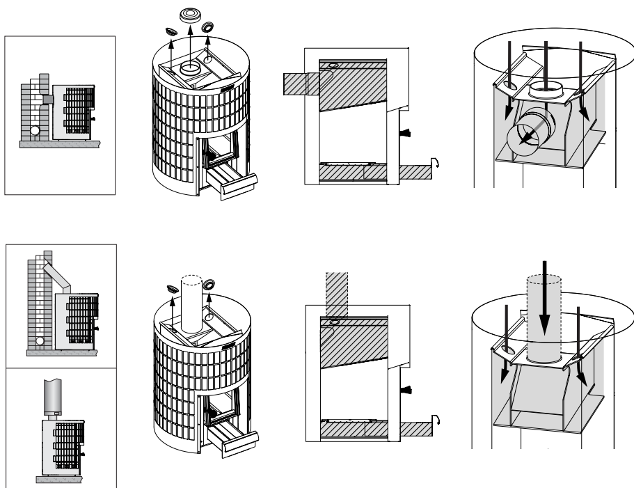
Рисунок 15. Чистка каменки
