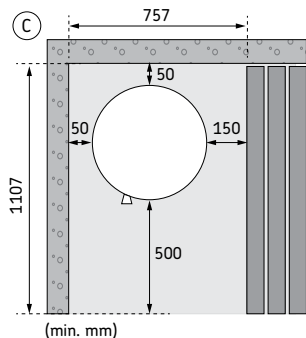
Kuva 6. Suojaetäisyydet
