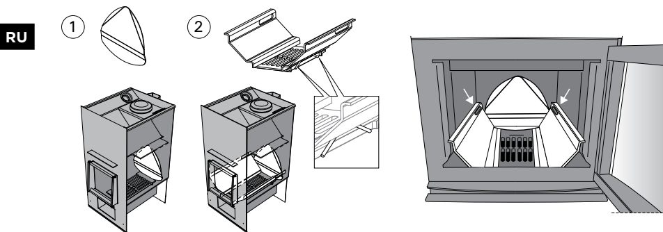
Рисунок 2. Дефлекторы топочного воздуха
