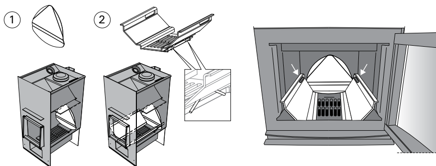
Kuva 2. Palamisilmanohjaimet
