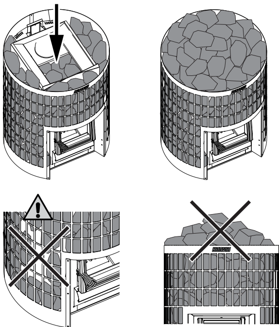
Kuva 13. Kiuaskivien latominen
