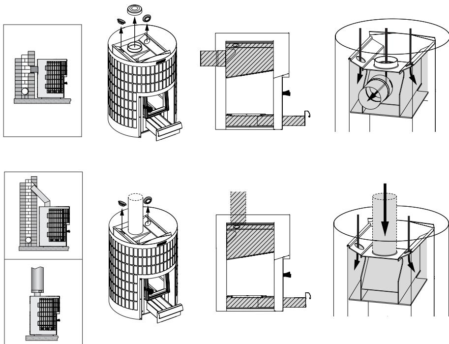
Kuva 15. Kiukaan nuohominen
